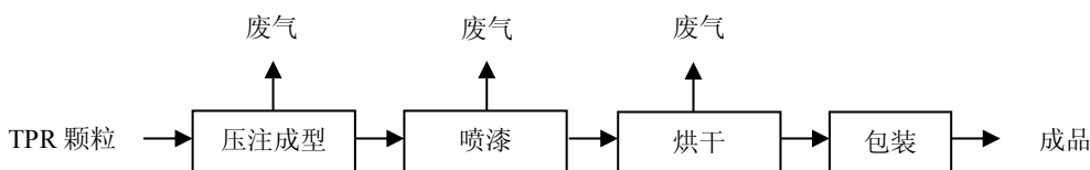
图 4-3 TPR 鞋底生产工艺
