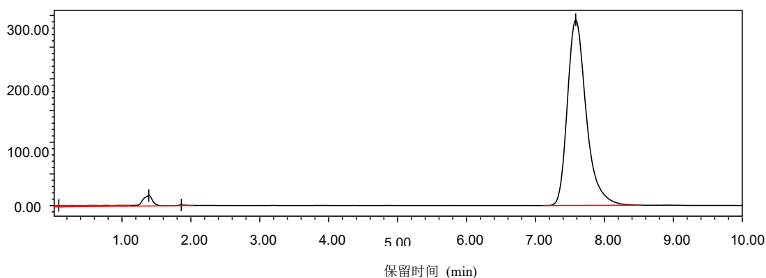
图 1 联苯胺标准色谱图 ( \rho = 50.0 \mu\text{g/L} )
